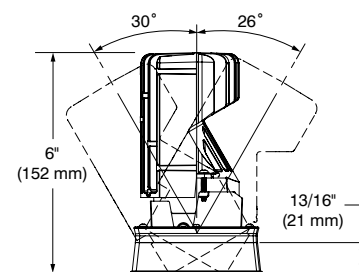
FLANGELESS TRIM
