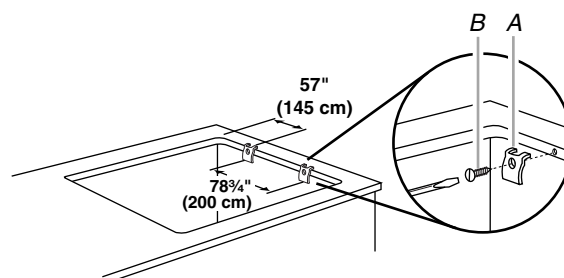
A. Attaches de montage
