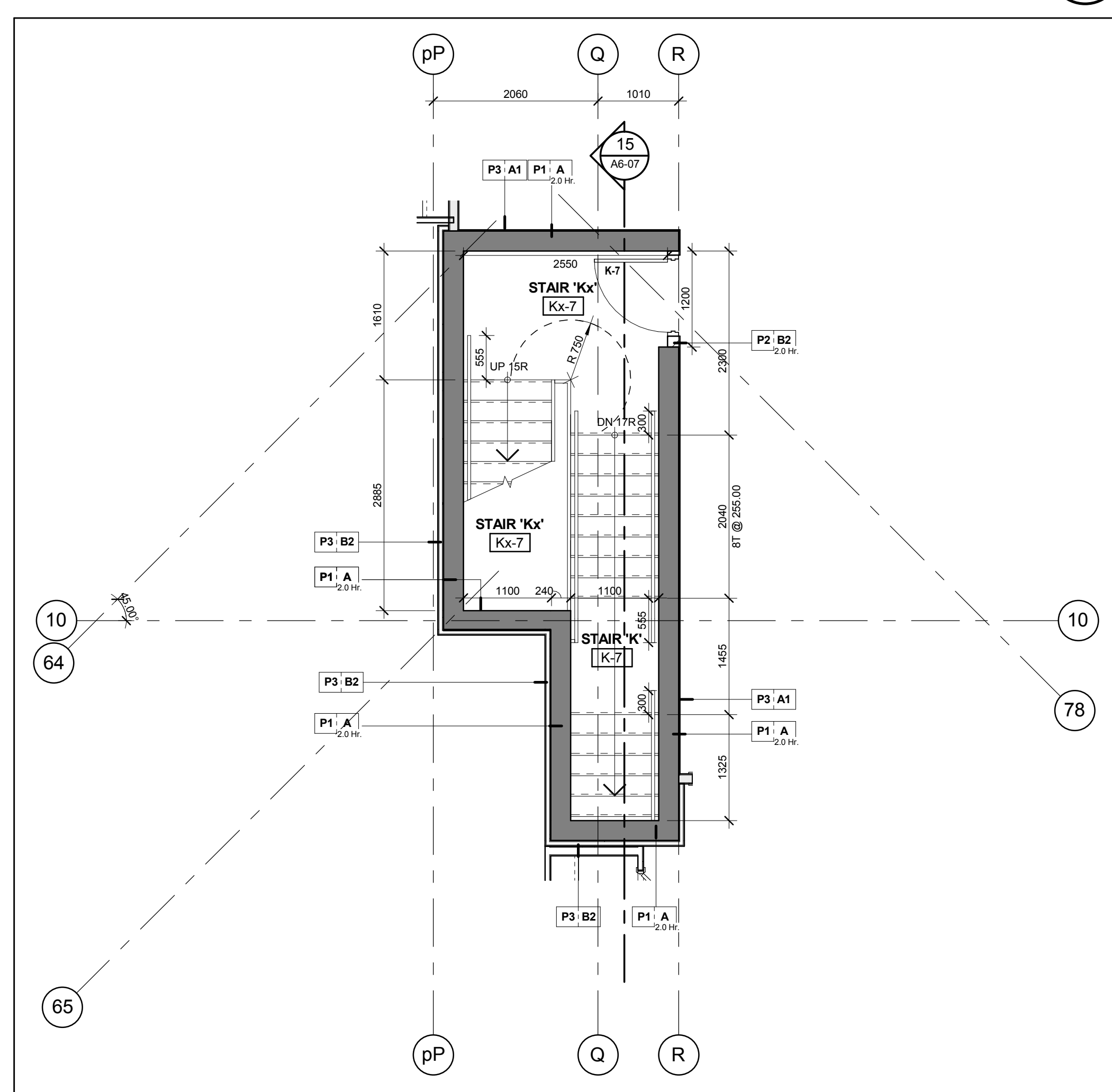
Stair 'K' & 'Kx' - Stair Plan - Level 7 Scale: 1 : 50
