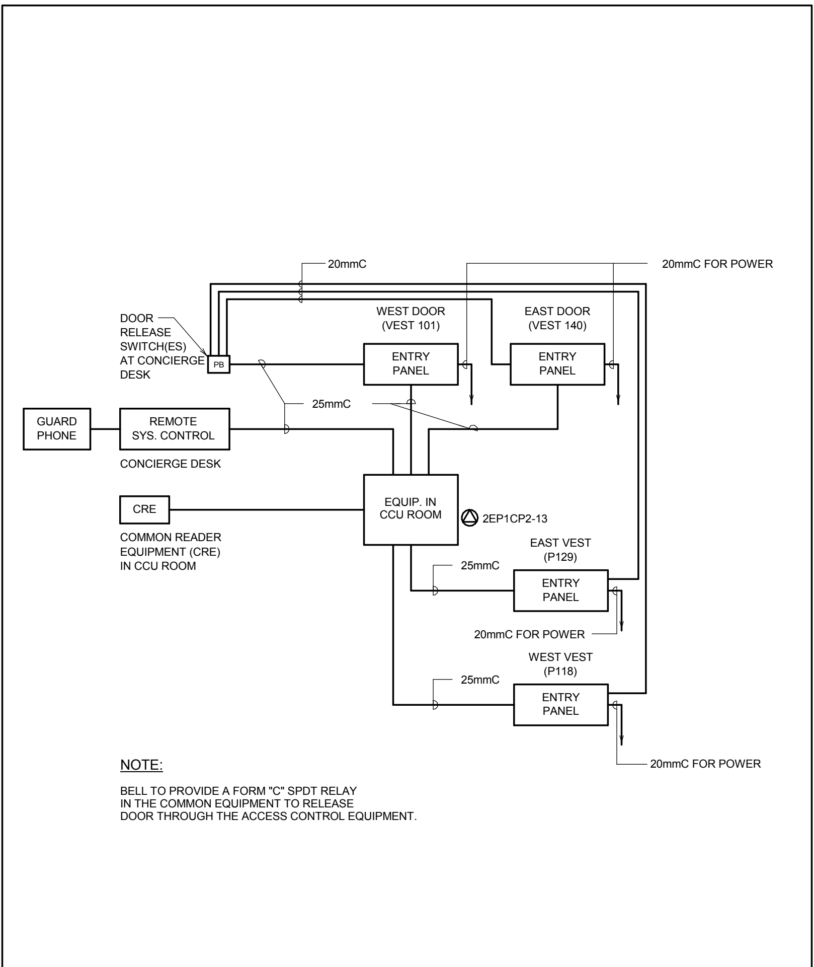
4 ENTERPHONE SYSTEM (CONDO) N.T.S.
