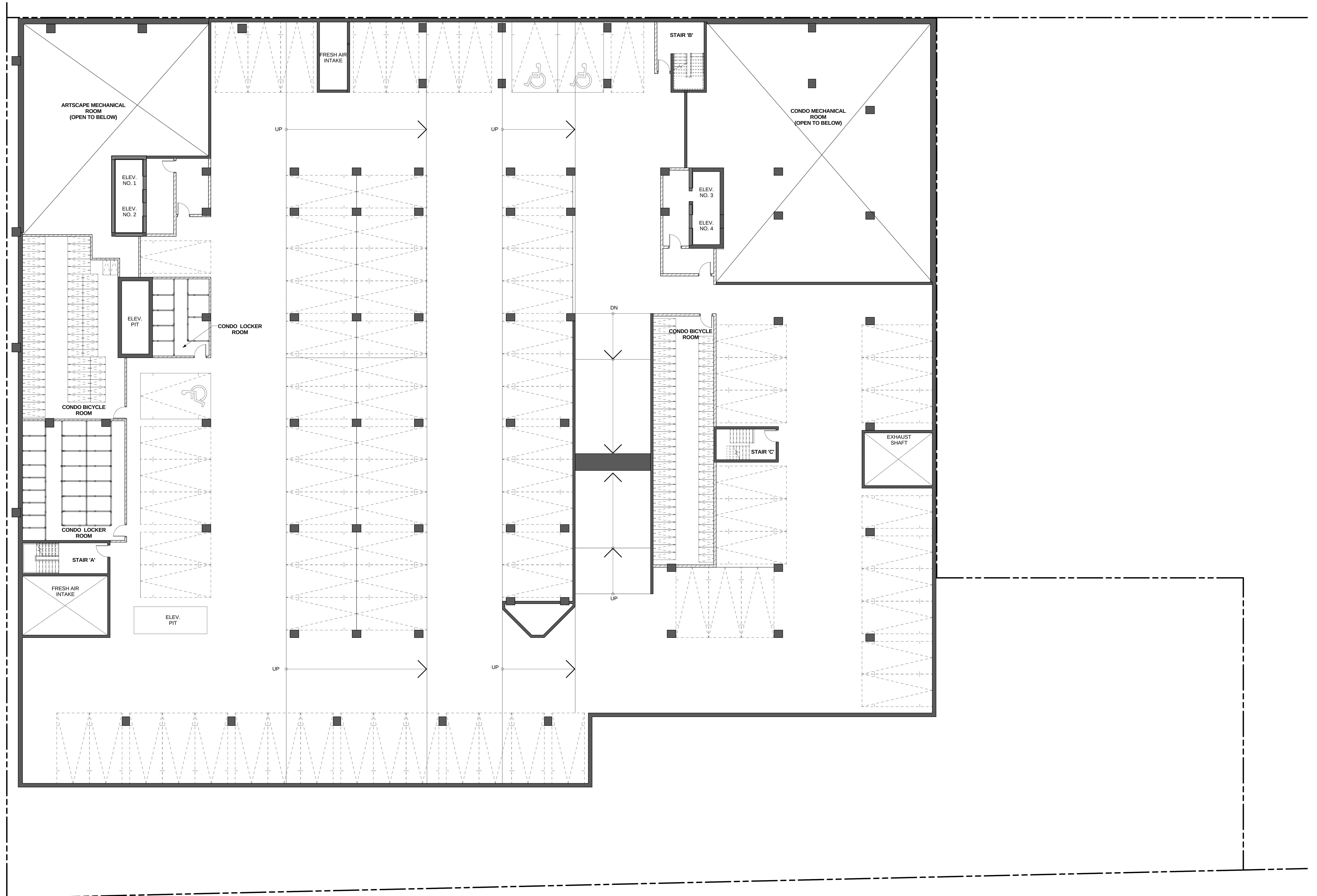
LEVEL P3 - 1:100
