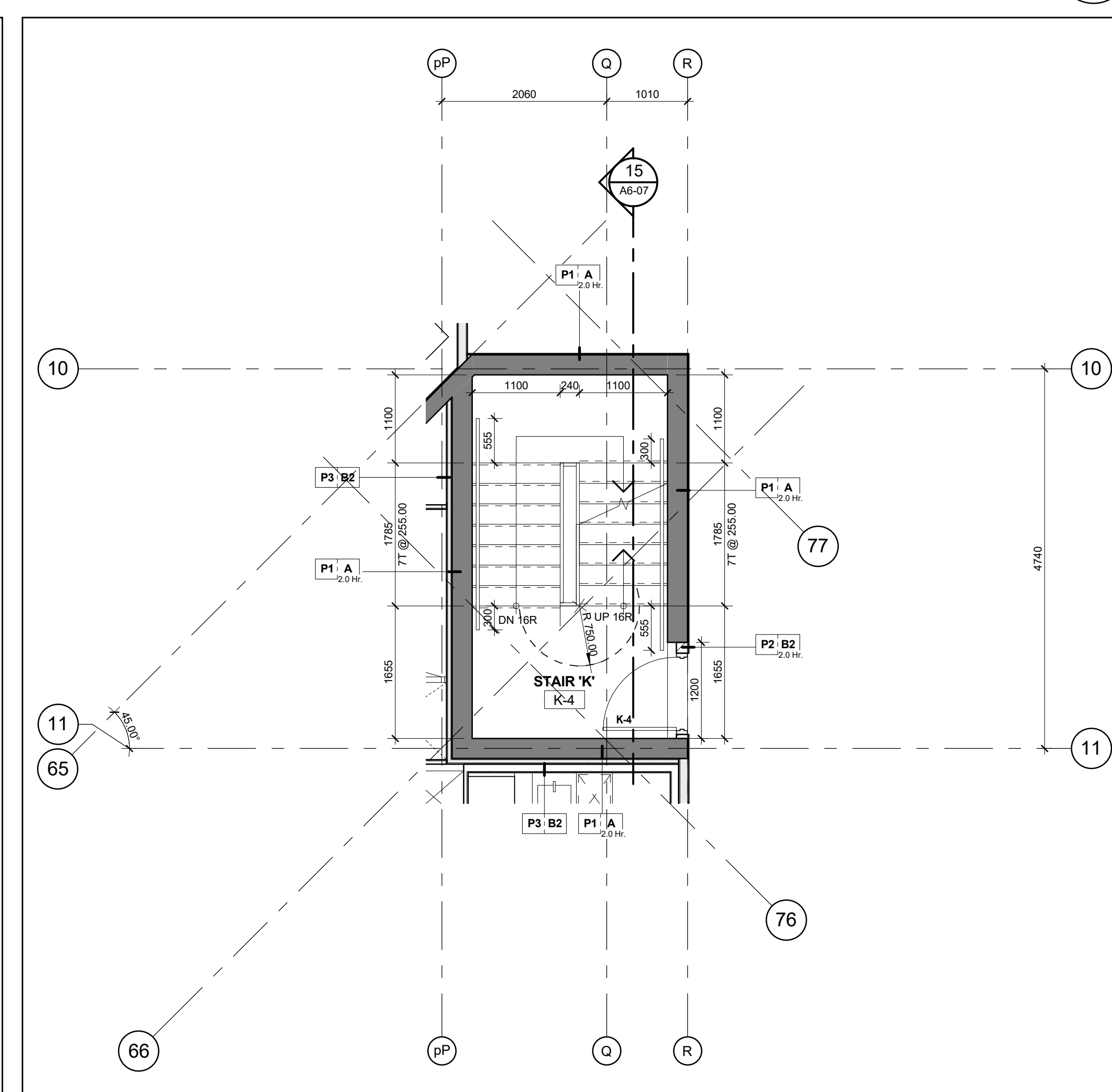
Stair 'K' - Stair Plan - Level 4 Scale: 1 : 50 A6-07
