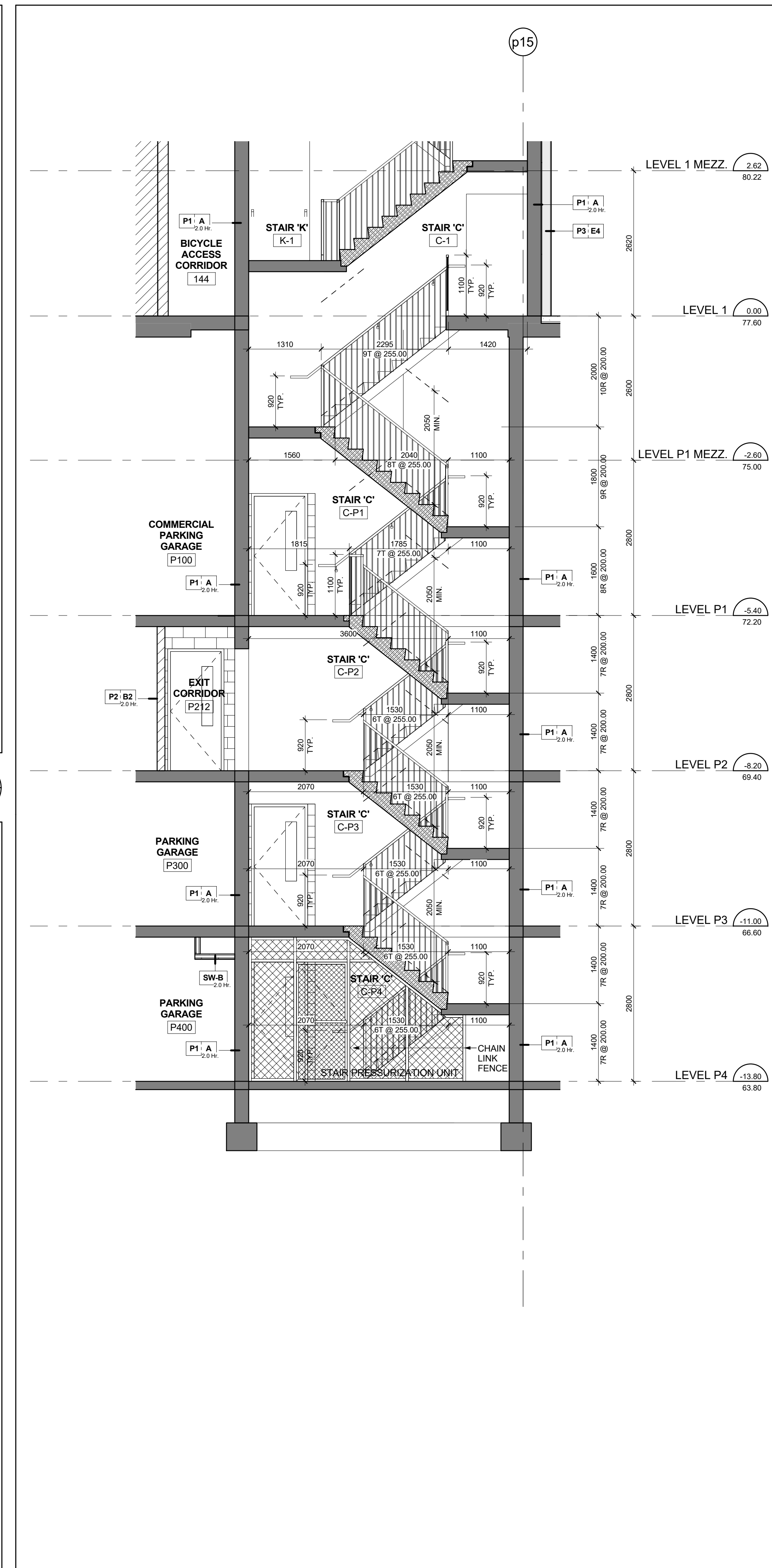
Stair 'C' - Stair Section Levels P4 - 1 Mezzanine Scale: 1 : 50
