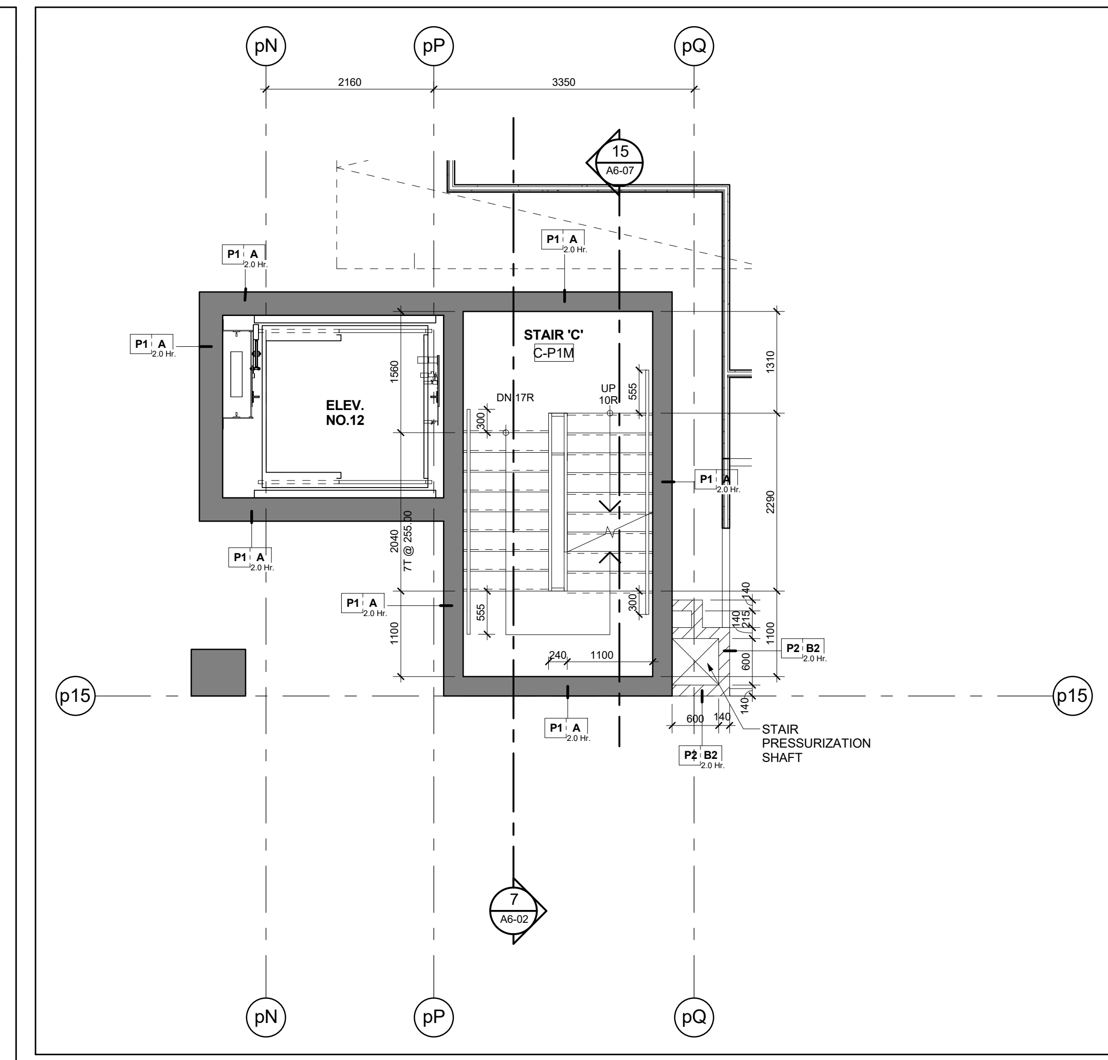
Stair 'C' - Stair Plan - Level P1 Mezzanine Scale: 1 : 50
