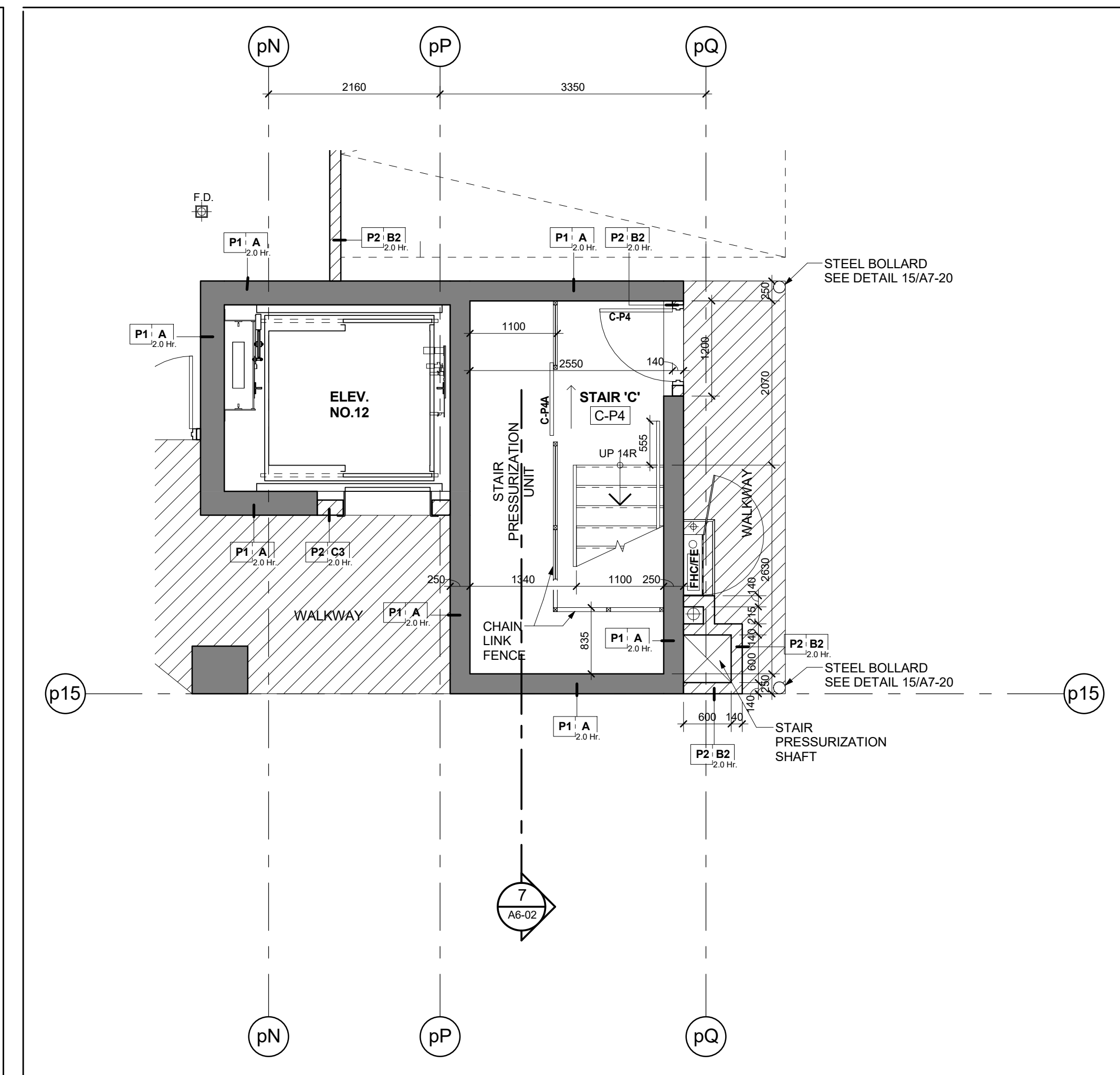
Stair 'C' - Stair Plan - Level P4 Scale: 1 : 50
