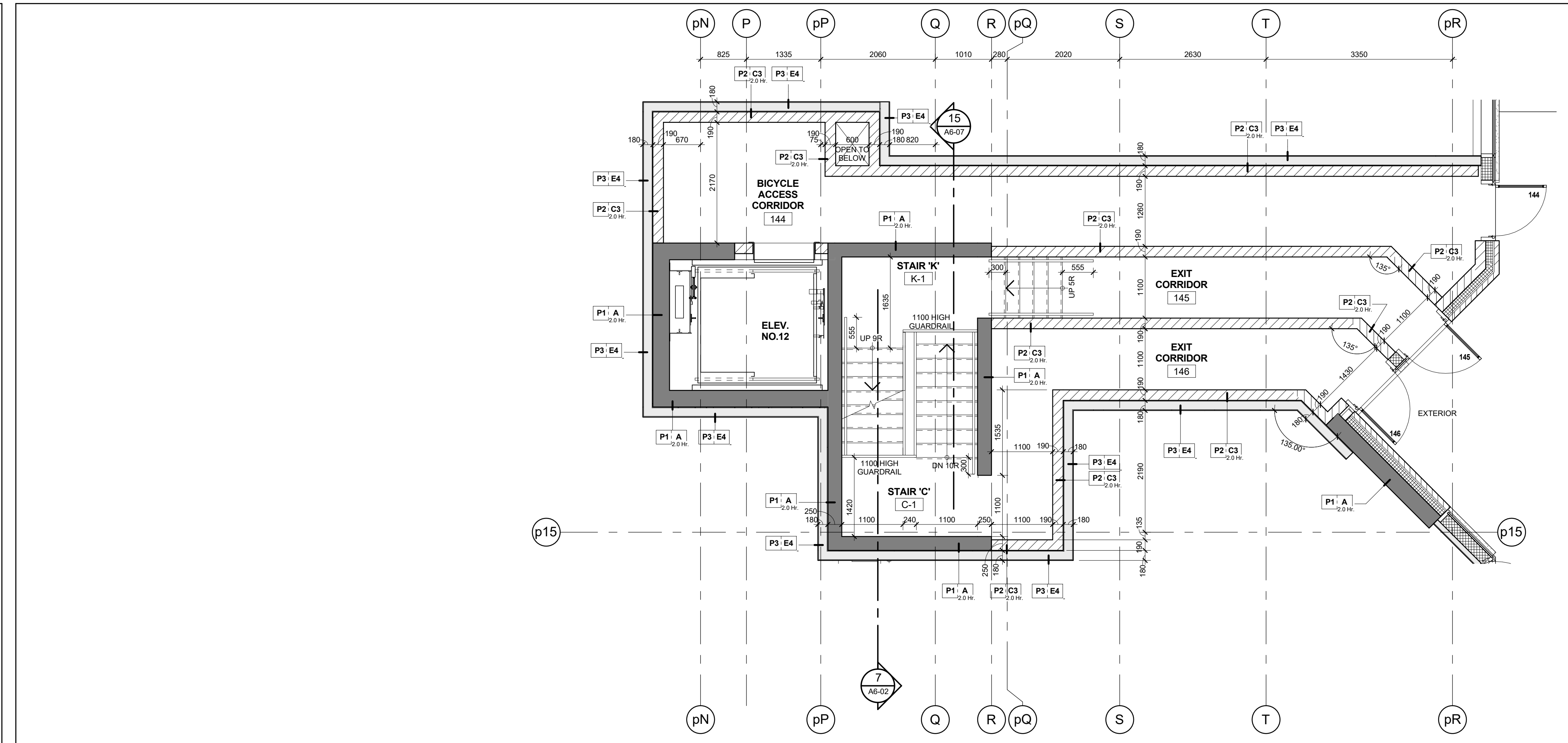
Stair 'C' - Stair Plan - Level 1 Scale: 1 : 50
