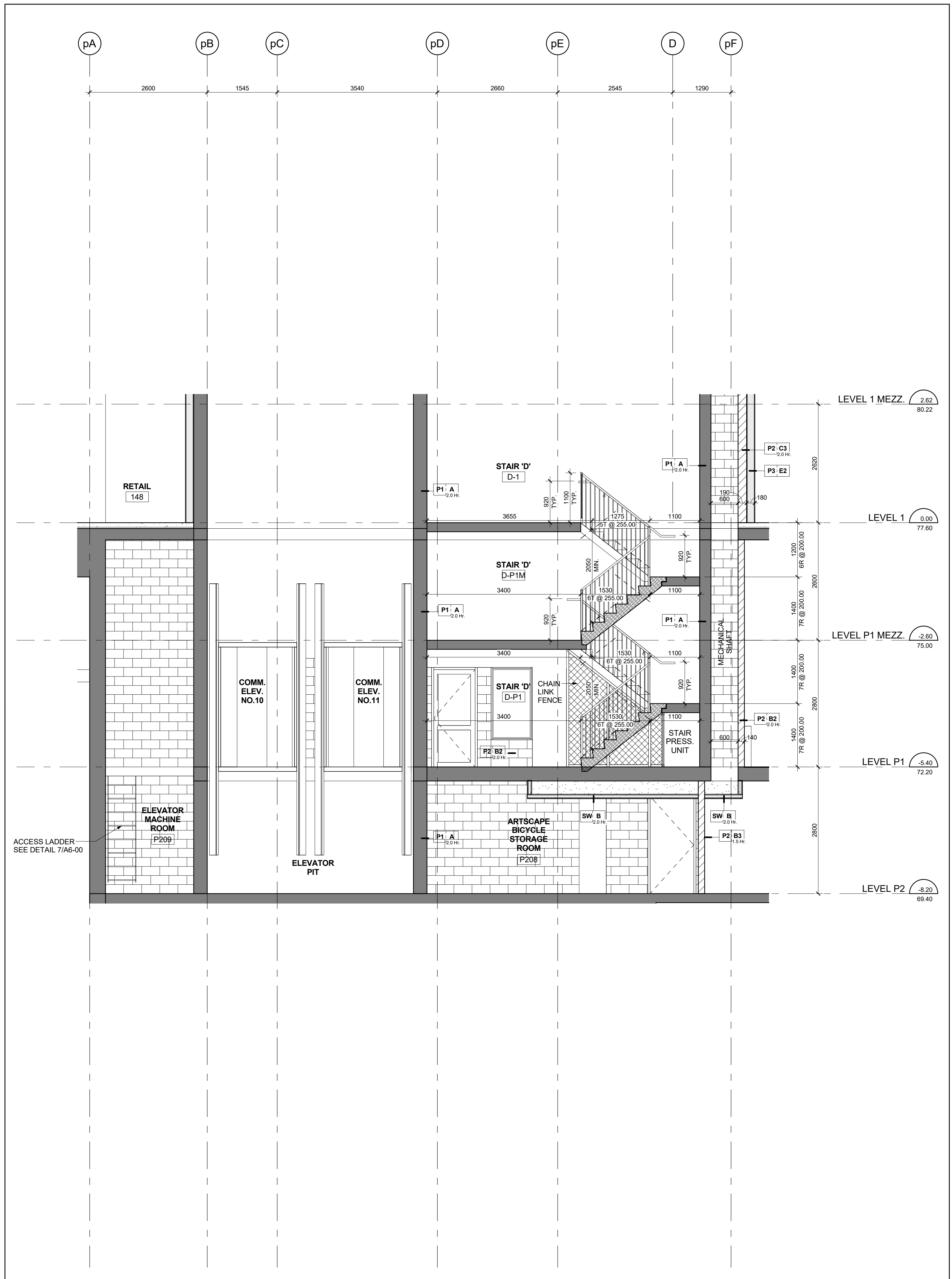
Stair 'D' - Stair Section - Levels P2 - 1 Mezzanine Scale: 1 : 50
