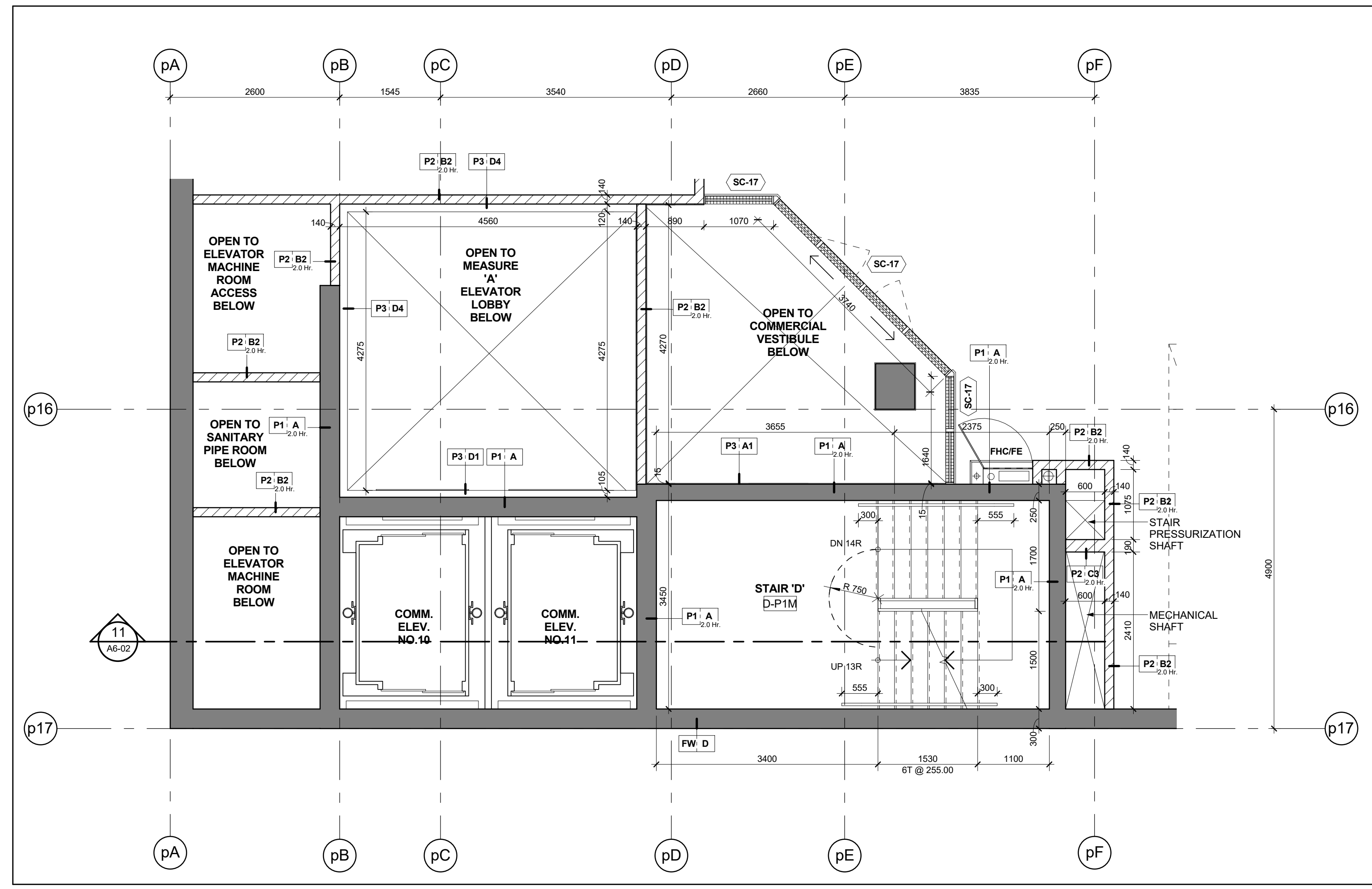
Stair 'D' - Stair Plan - Level P1 Mezzanine Scale: 1 : 50
