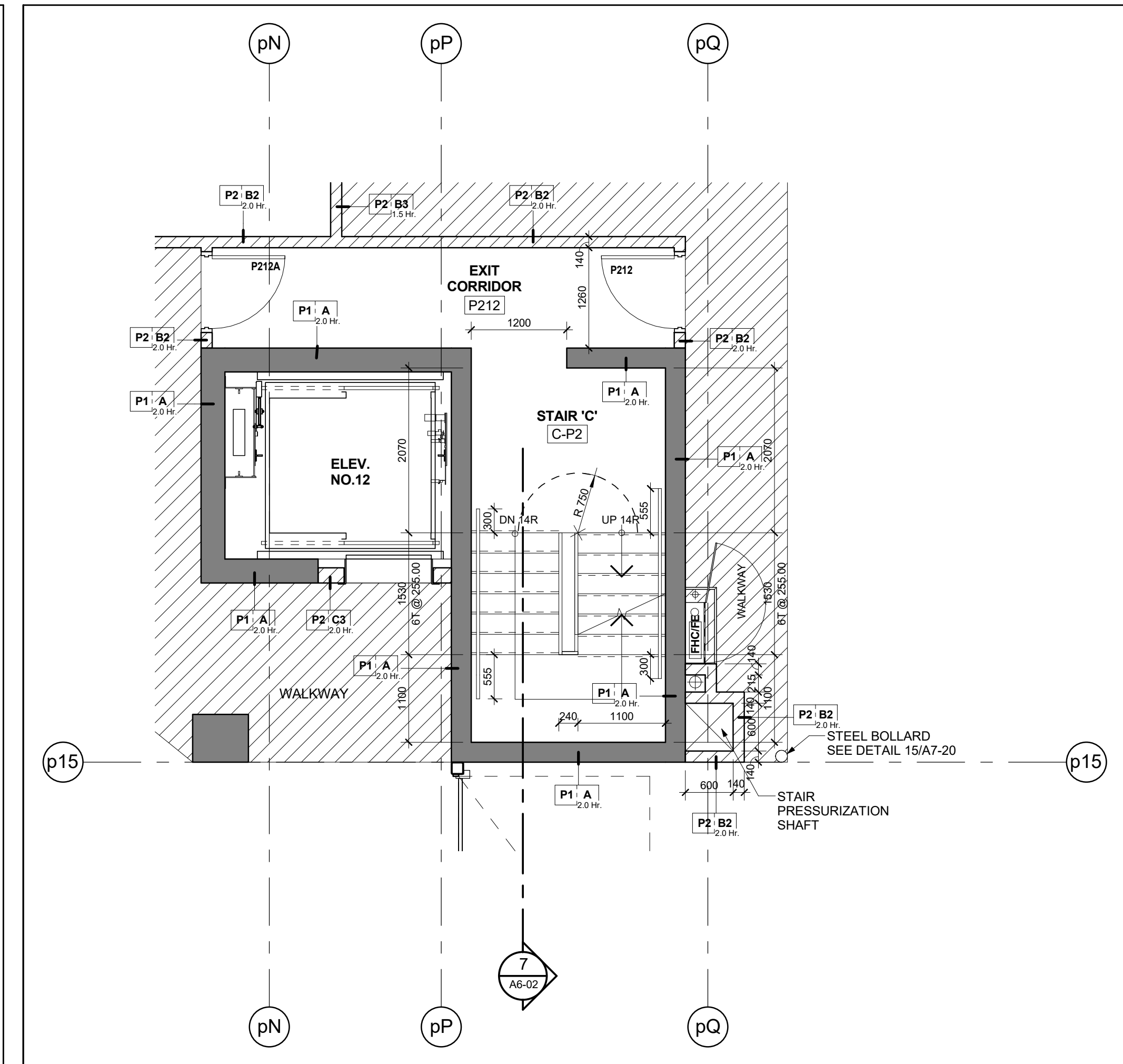
Stair 'C' - Stair Plan - Level P2 Scale: 1 : 50
