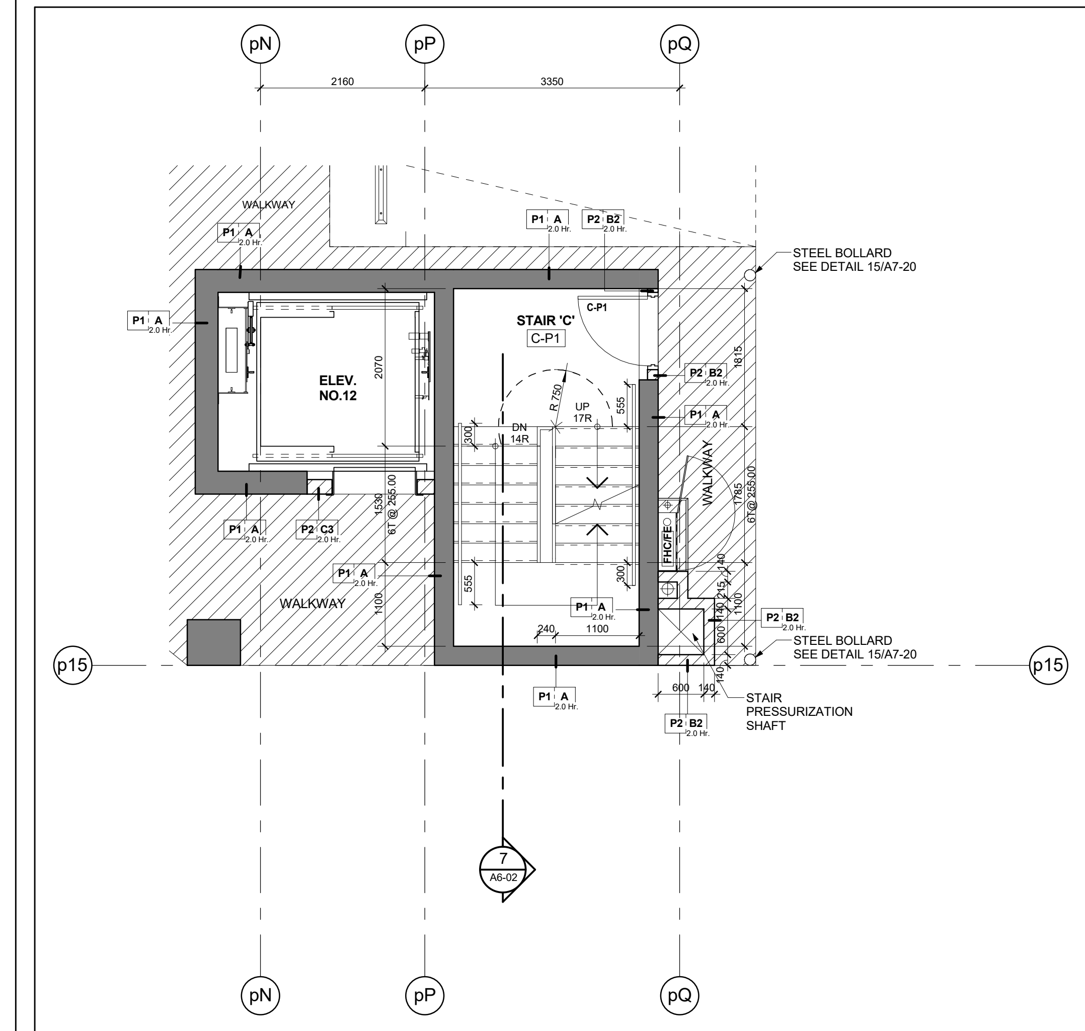
Stair 'C' - Stair Plan - Level P1 Scale: 1 : 50
