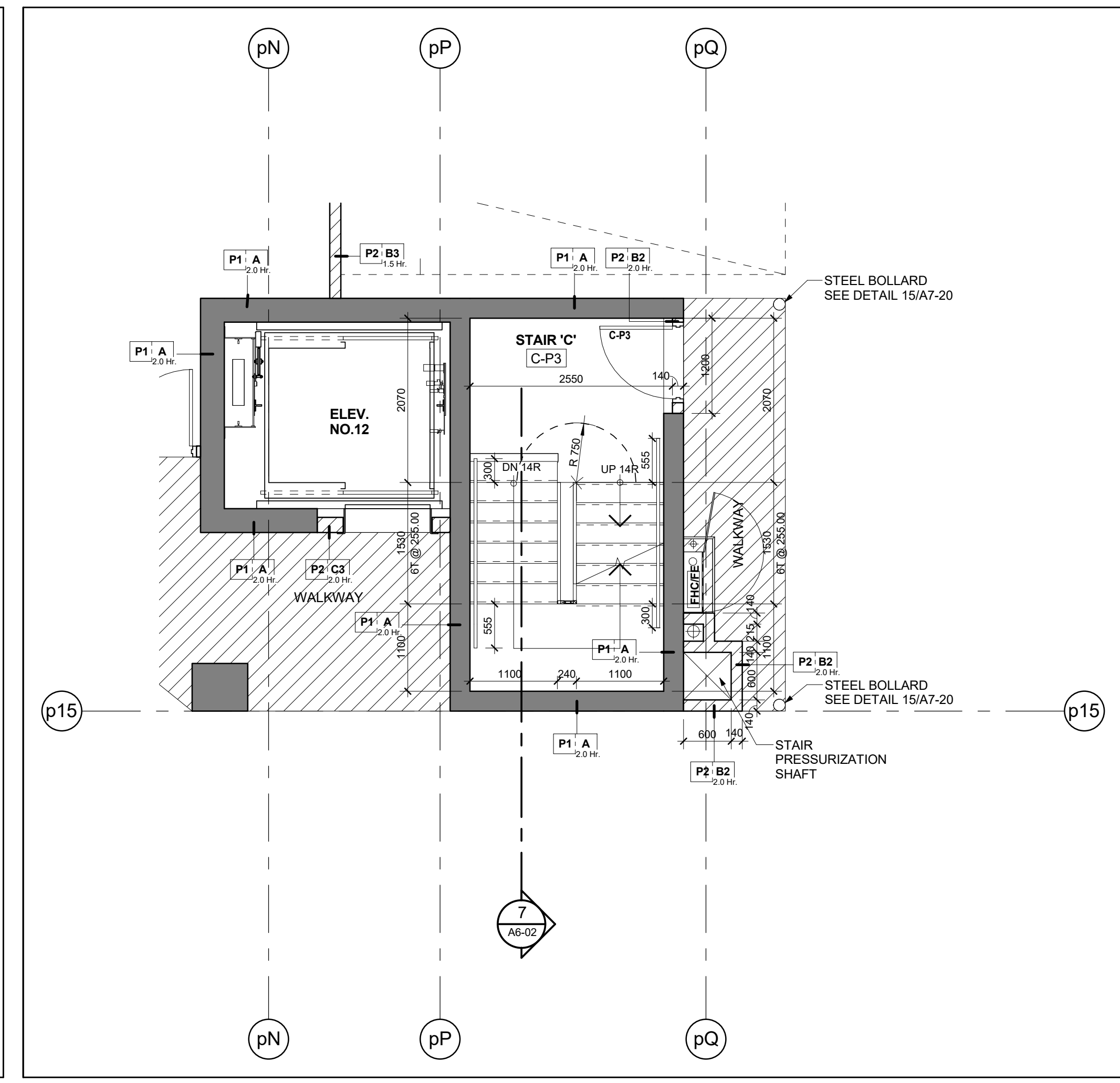
Stair 'C' - Stair Plan - Level P3 Scale: 1 : 50
