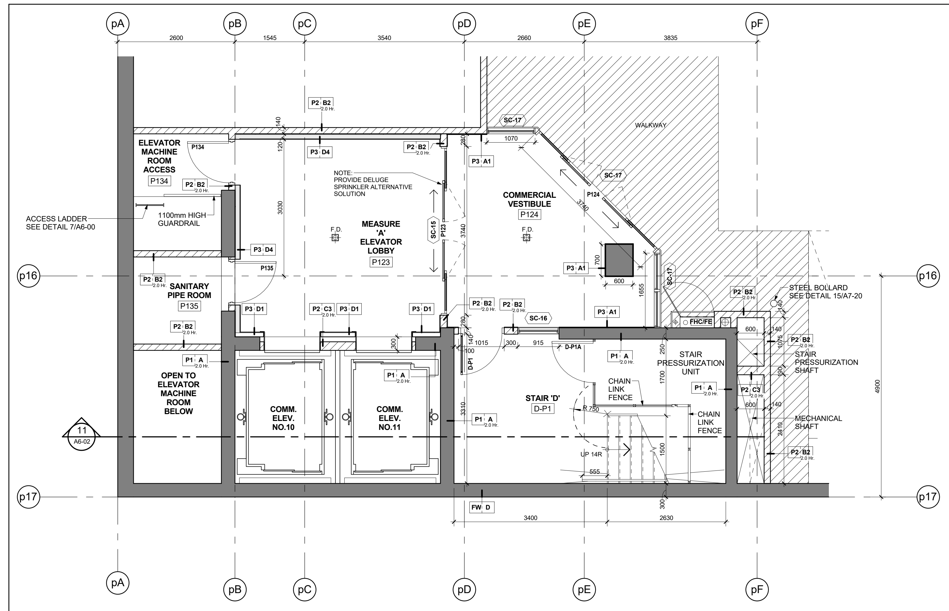
Stair 'D' - Stair Plan - Level P1 Scale: 1 : 50
