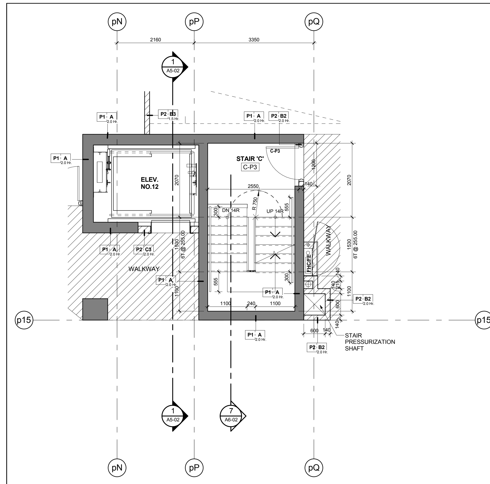
Stair 'C' - Stair Plan - Level P3 Scale: 1 : 50
