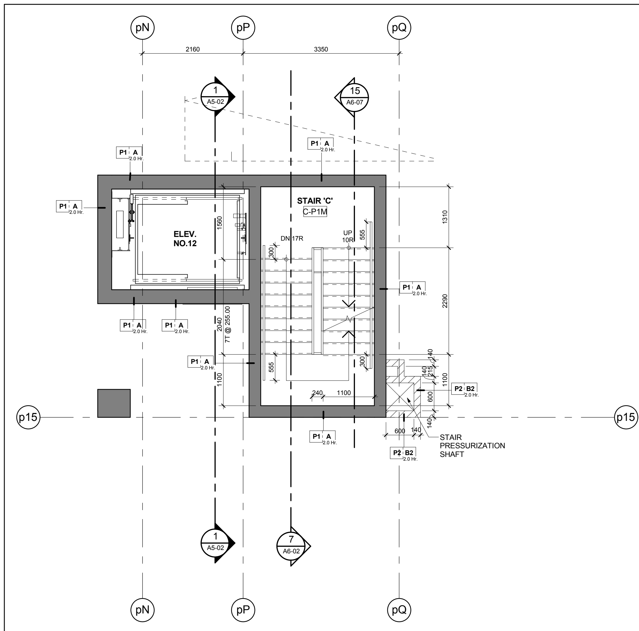
Stair 'C' - Stair Plan - Level P1 Mezzanine Scale: 1 : 50
