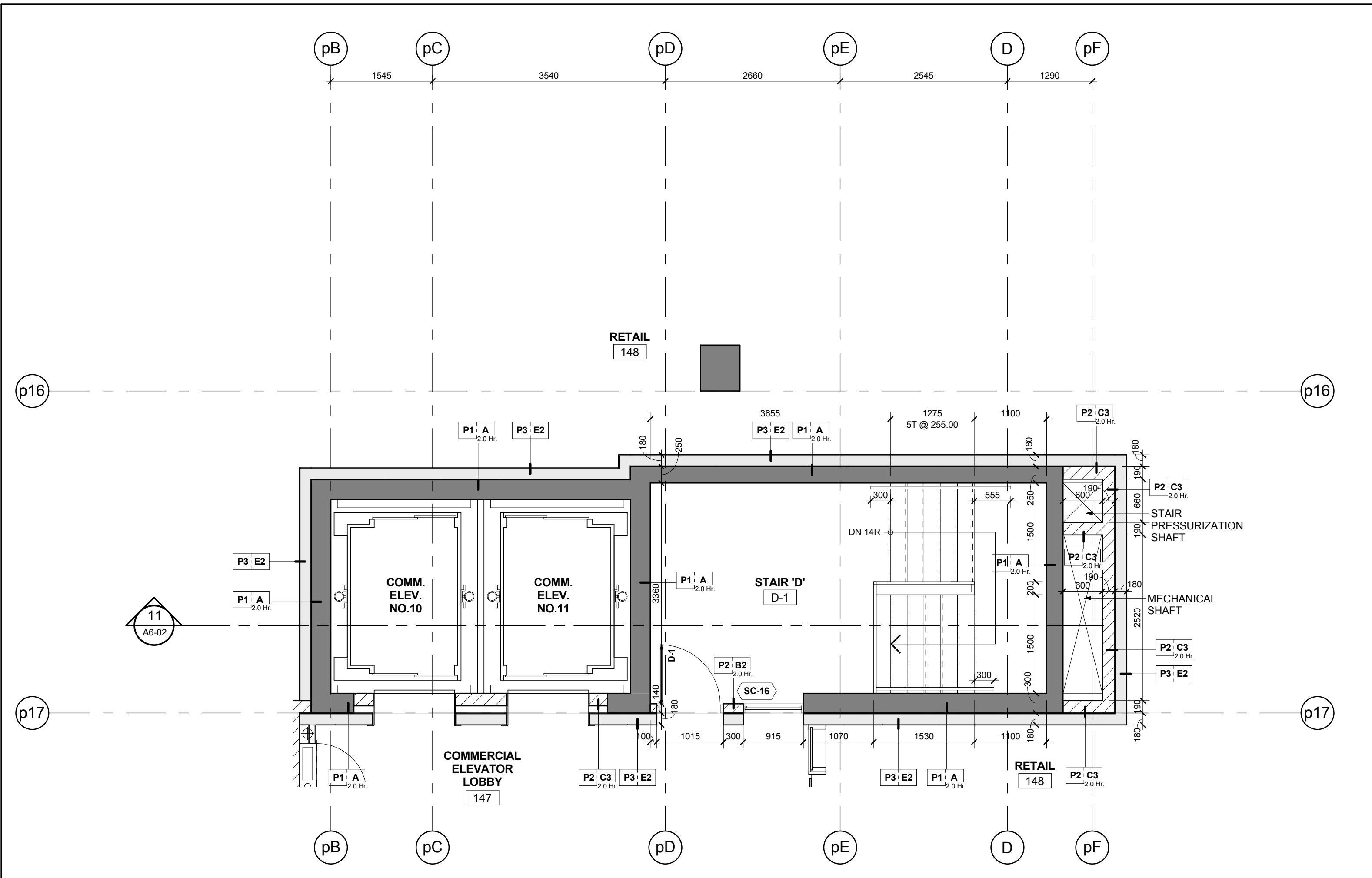
Stair 'D' - Stair Plan - Level 1 Scale: 1 : 50
