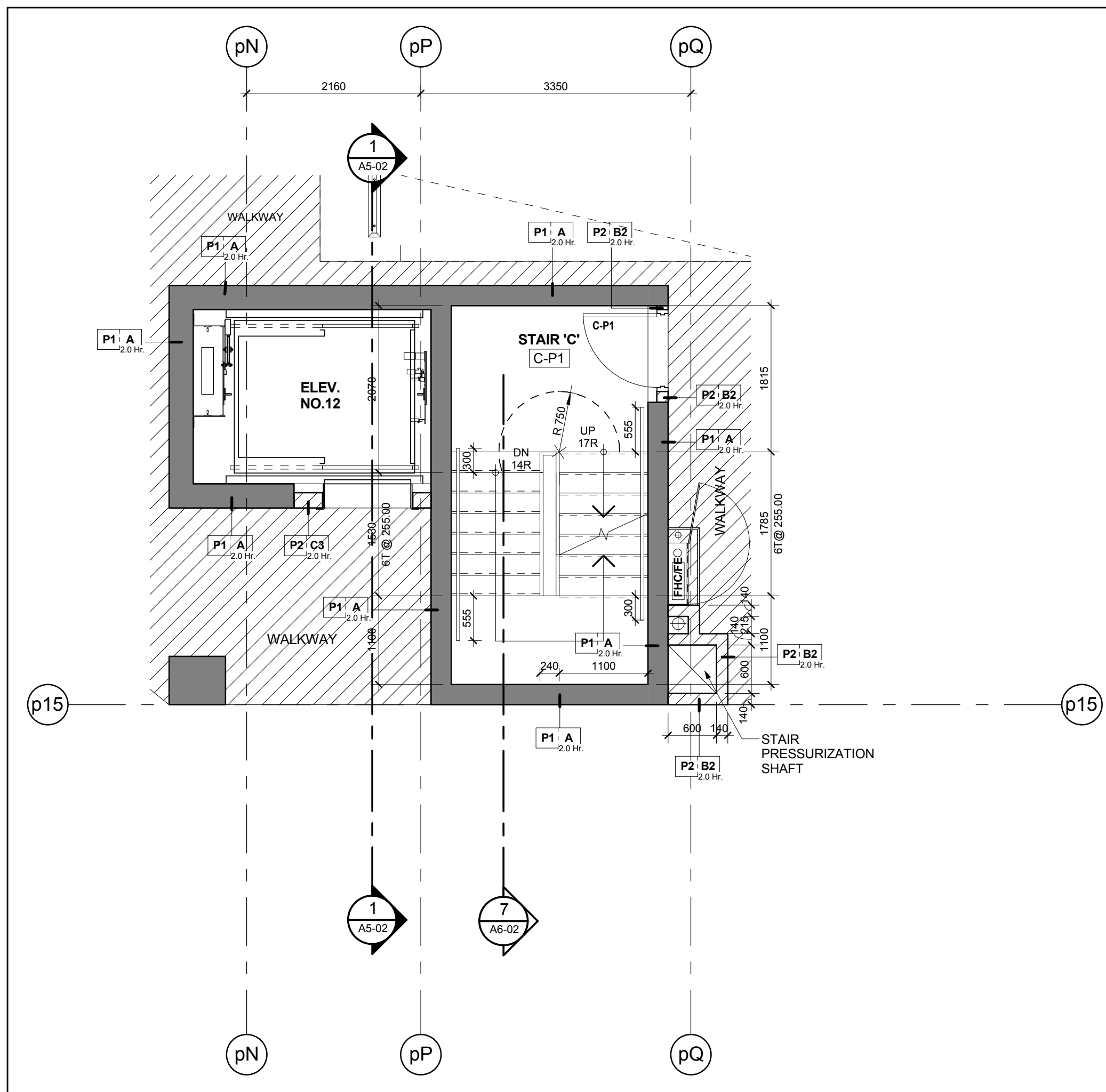
Stair 'C' - Stair Plan - Level P1 Scale: 1 : 50
