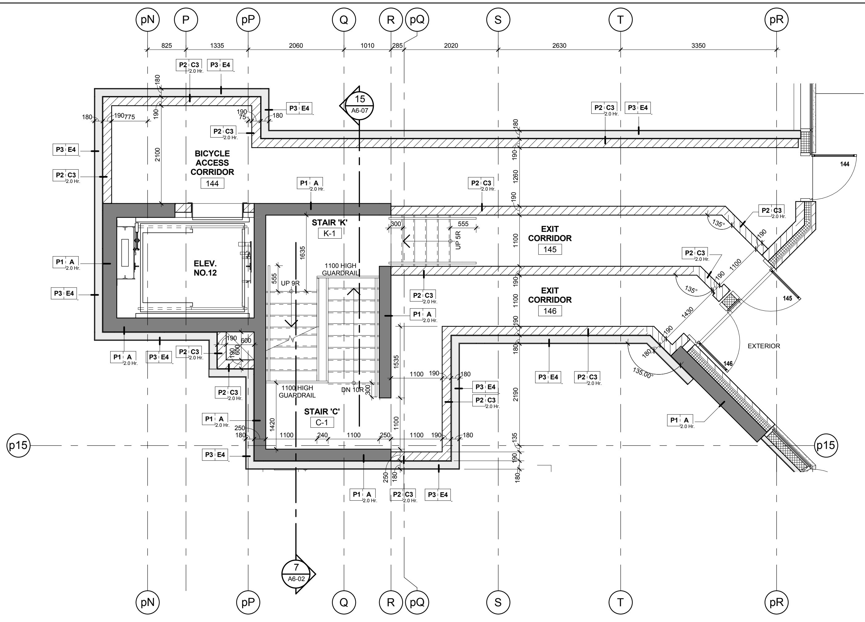
Stair 'C' - Stair Plan - Level 1 Scale: 1 : 50
