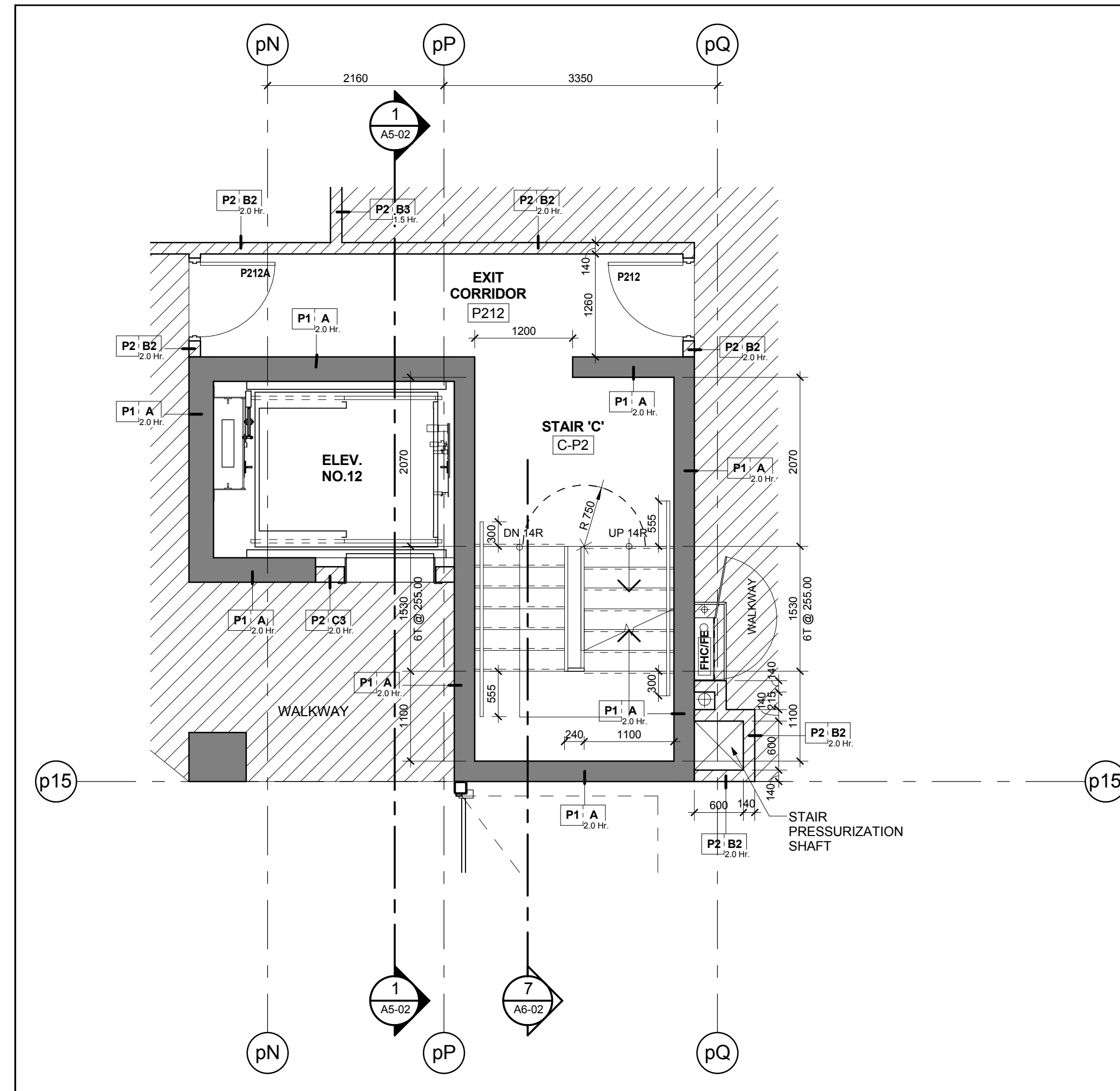
Stair 'C' - Stair Plan - Level P2 Scale: 1 : 50
