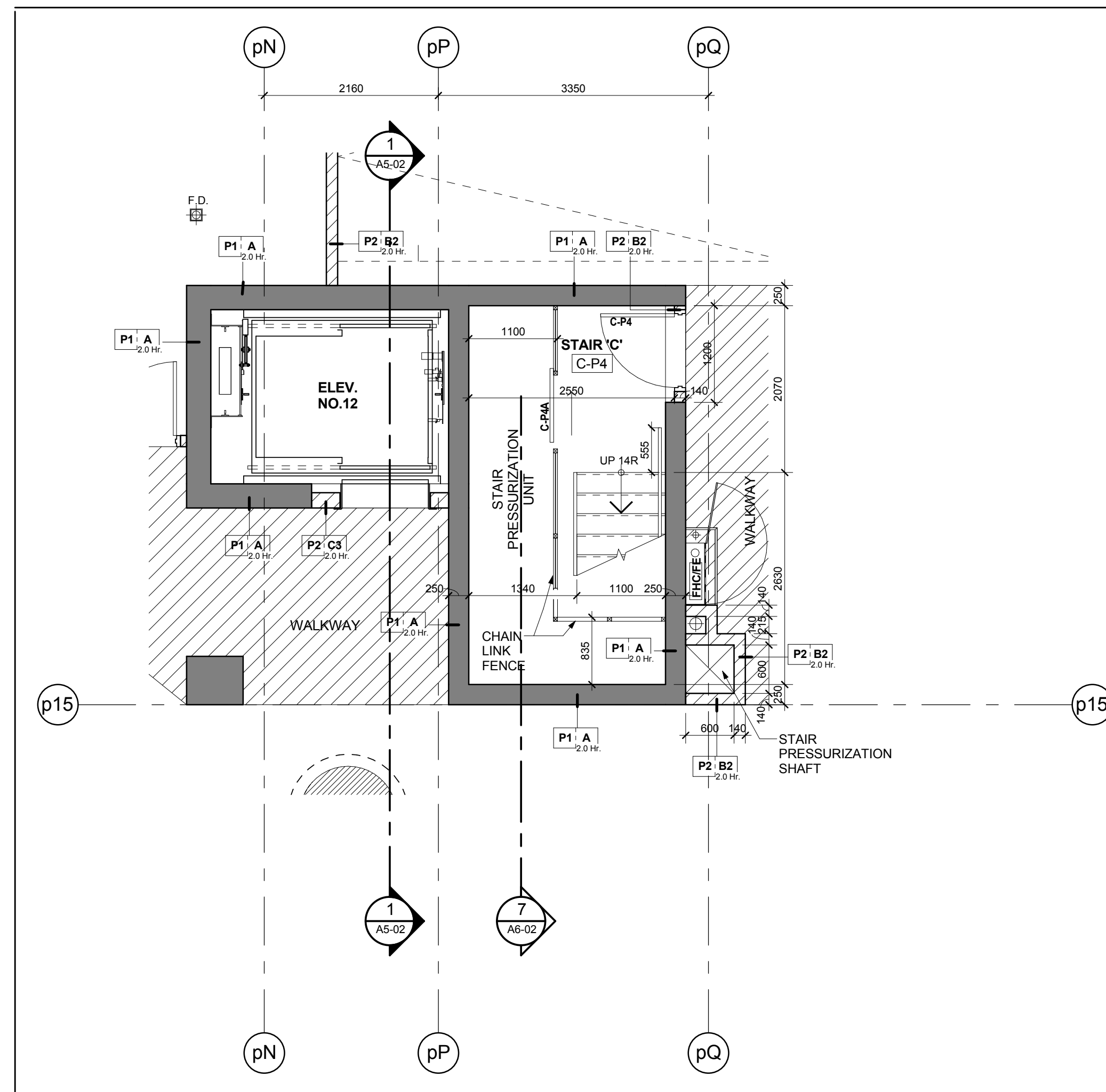
Stair 'C' - Stair Plan - Level P4 Scale: 1 : 50
