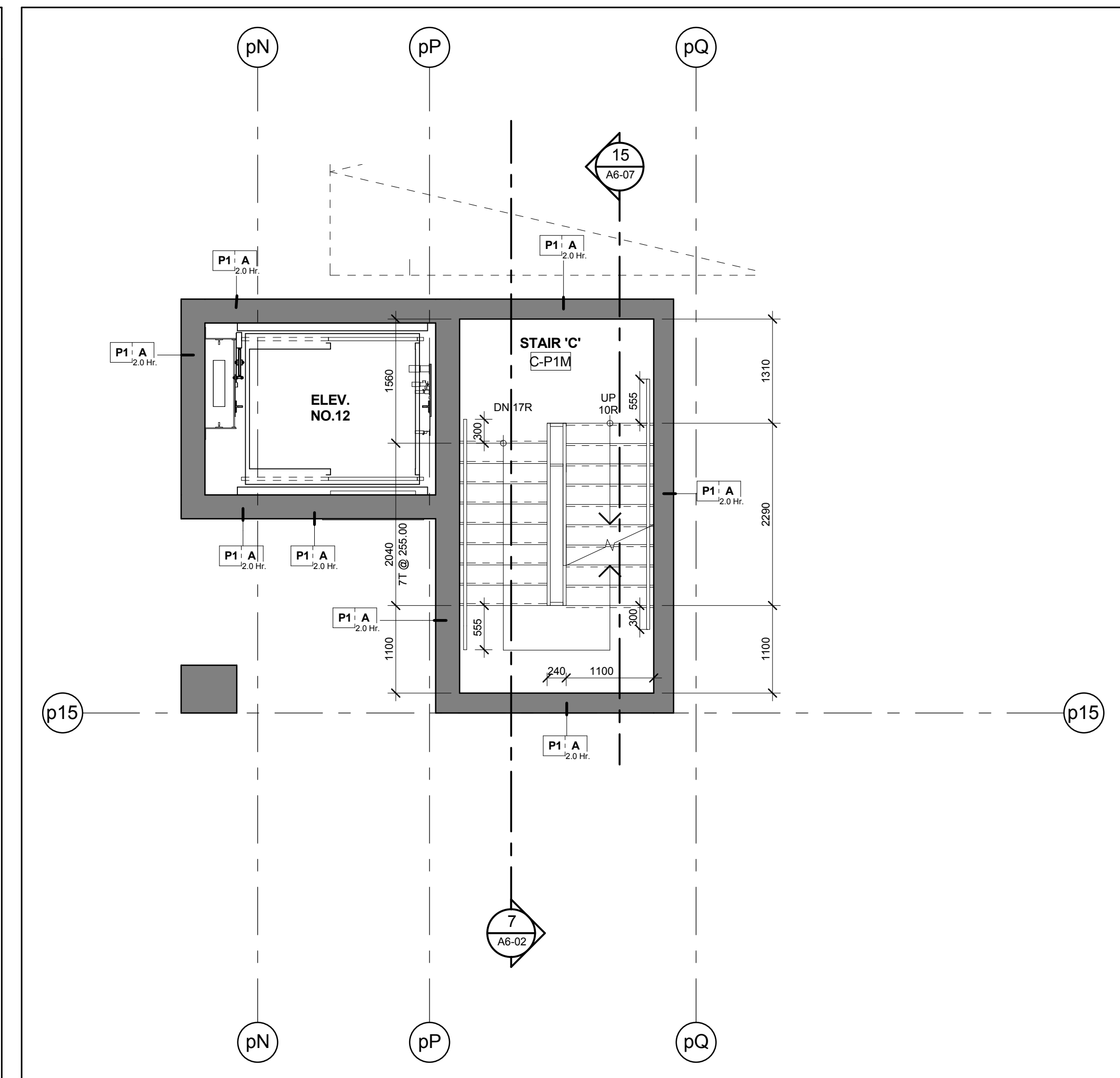
Stair 'C' - Stair Plan - Level P1 Mezzanine Scale: 1 : 50 A6-02
