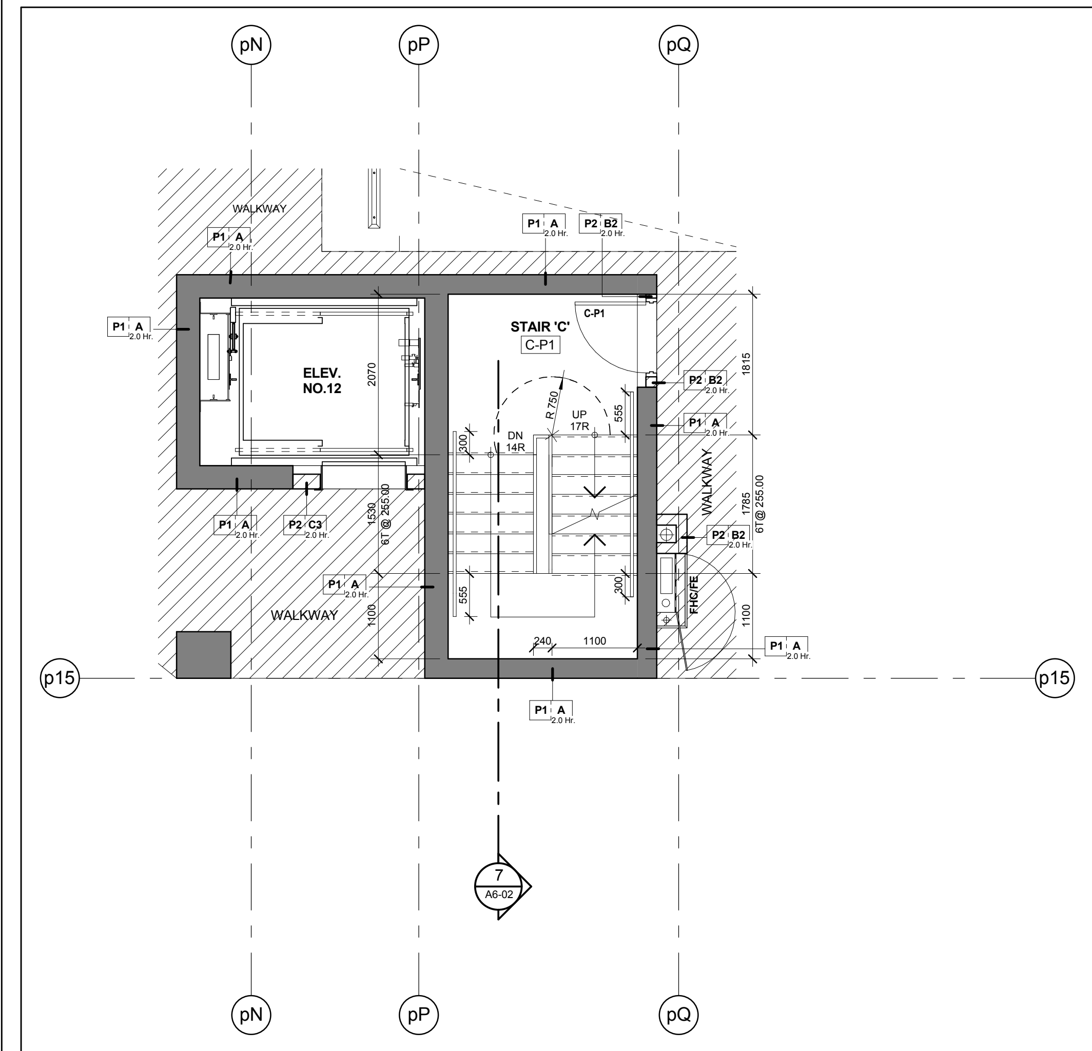
Stair 'C' - Stair Plan - Level P1 Scale: 1 : 50 A6-02
