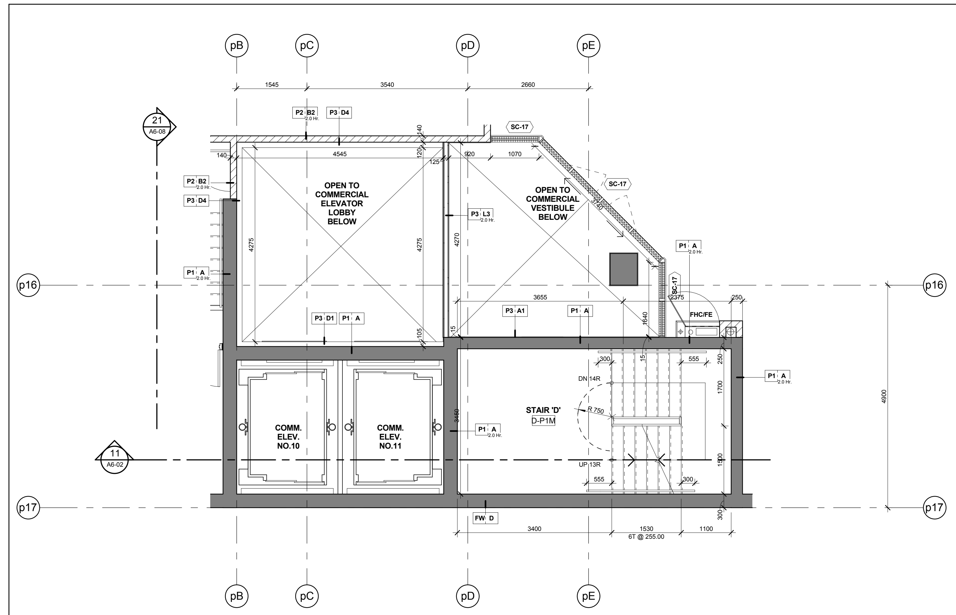
Stair 'D' - Stair Plan - Level P1 Mezzanine Scale: 1 : 50 A6-02
