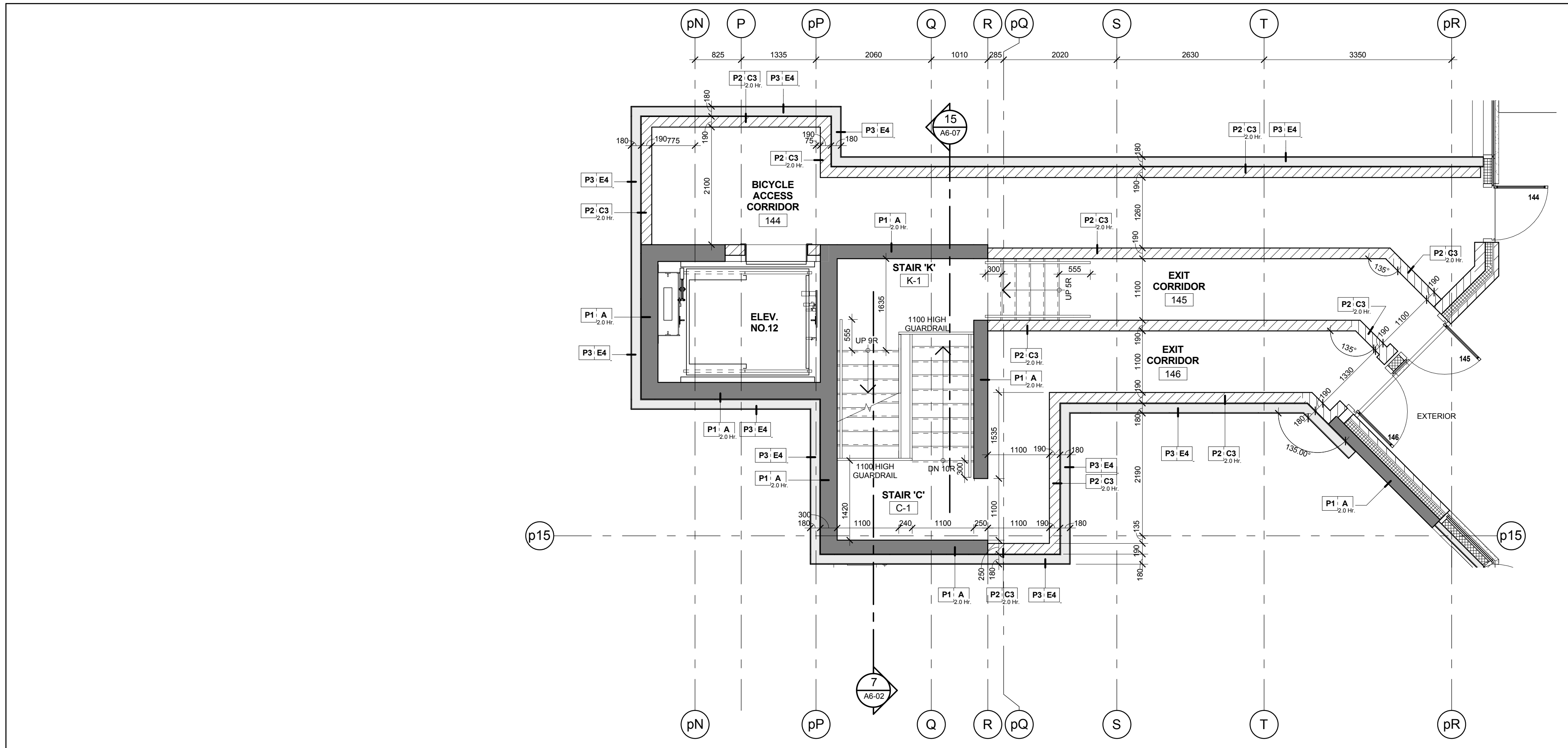
Stair 'C' - Stair Plan - Level 1 Scale: 1 : 50 A6-02
