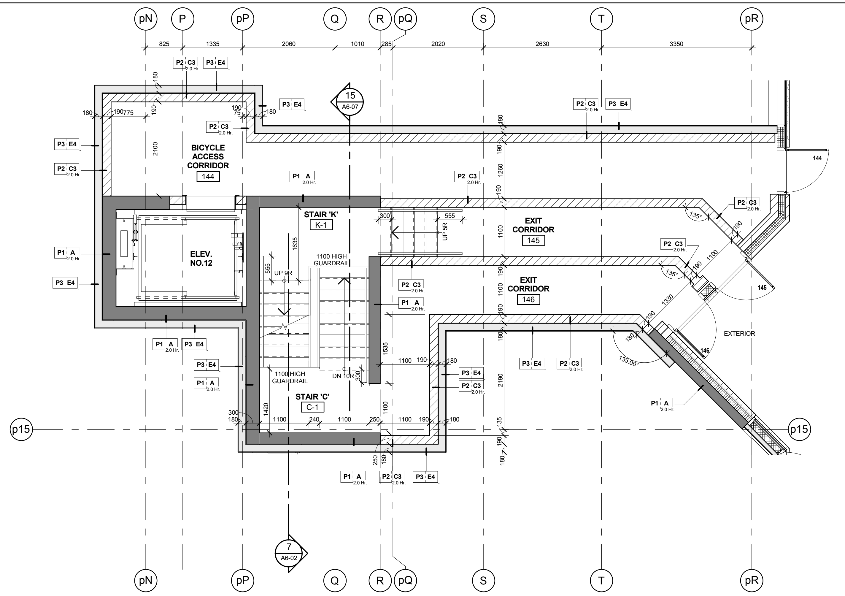
Stair 'C' - Stair Plan - Level 1 Scale: 1 : 50
