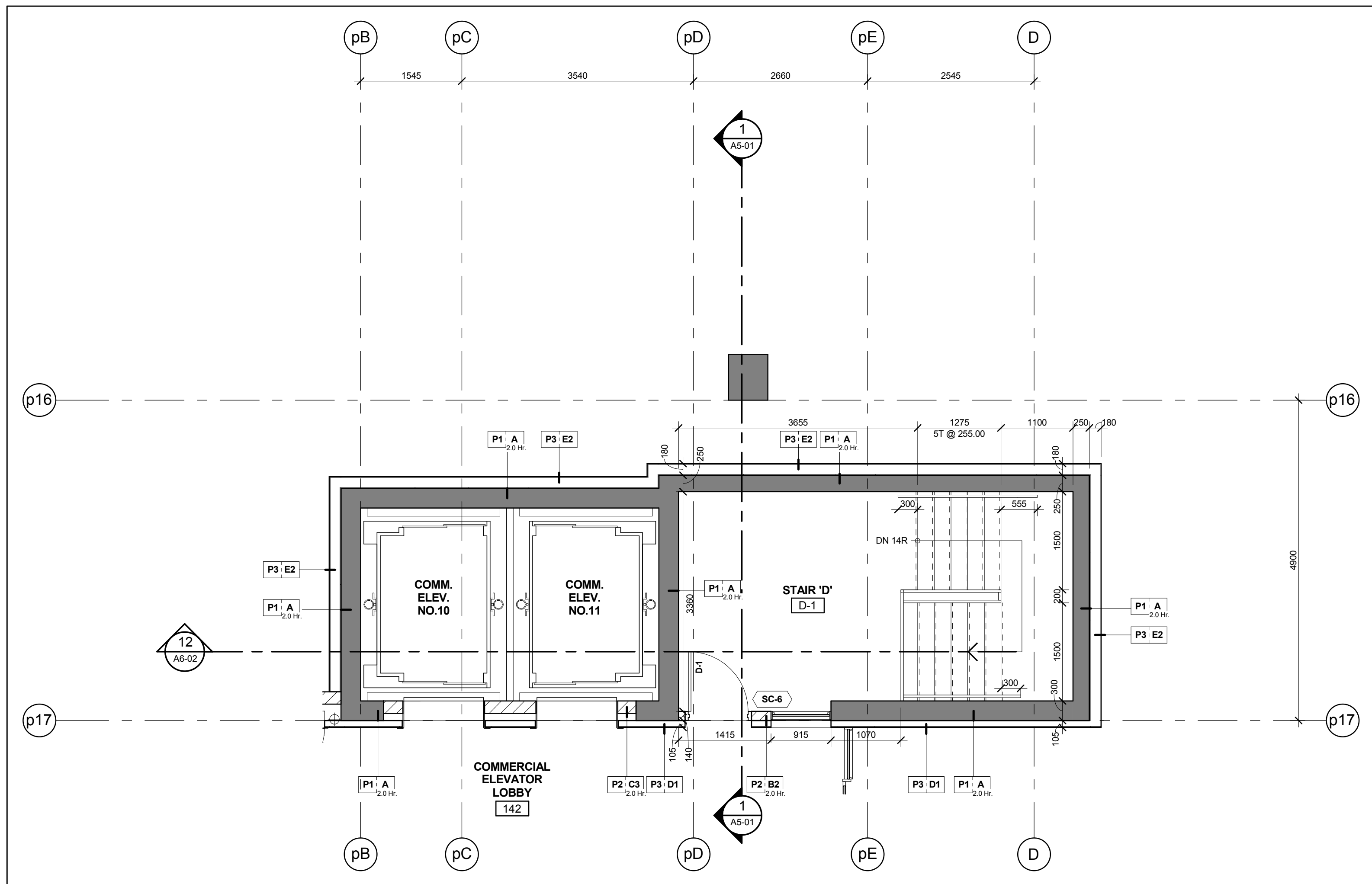
Stair 'D' - Stair Plan - Level 1 Scale: 1 : 50 A6-02
