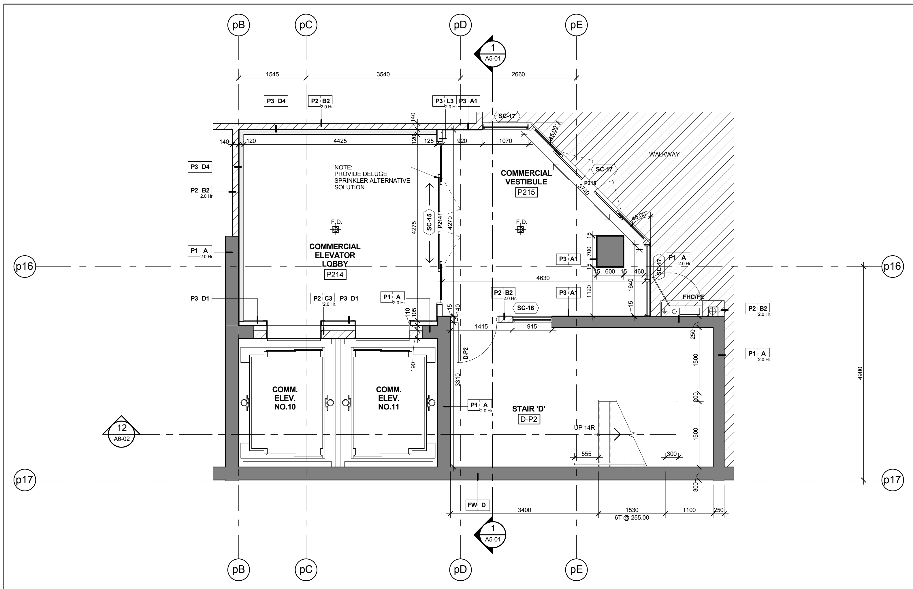
Stair 'D' - Stair Plan - Level P2 Scale: 1 : 50 A6-02
