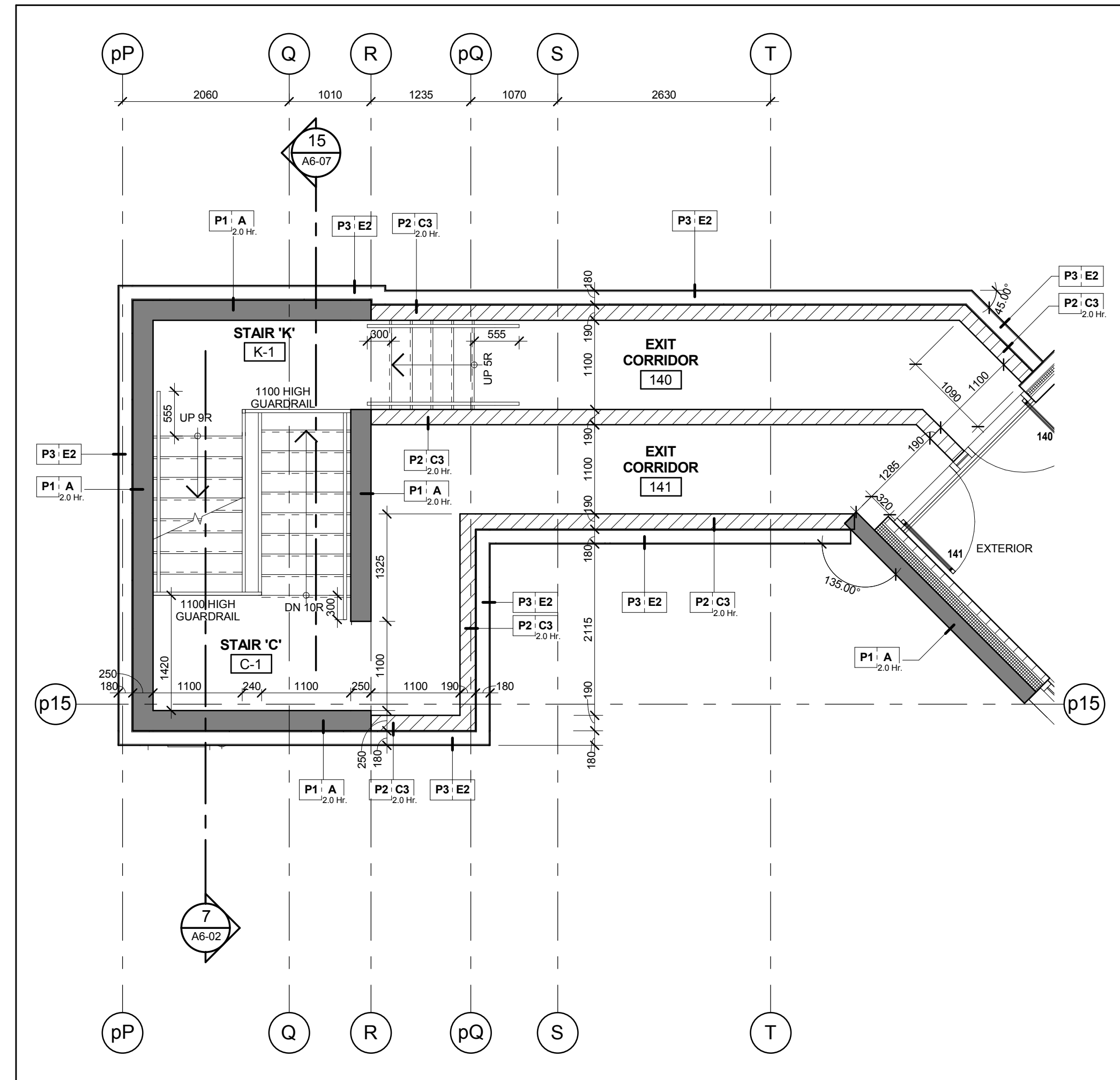
Stair 'C' - Stair Plan - Level 1 Scale: 1 : 50 A6-02
