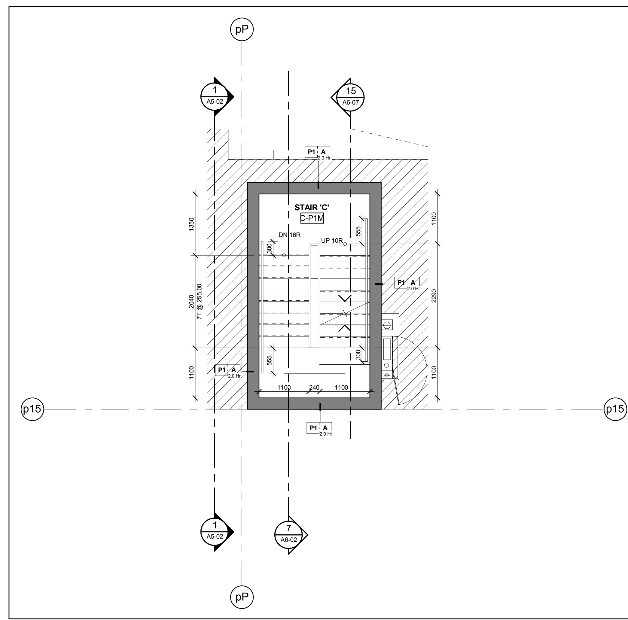
Stair 'C' - Stair Plan - Level P1 Mezzanine Scale: 1 : 50 A6-02
