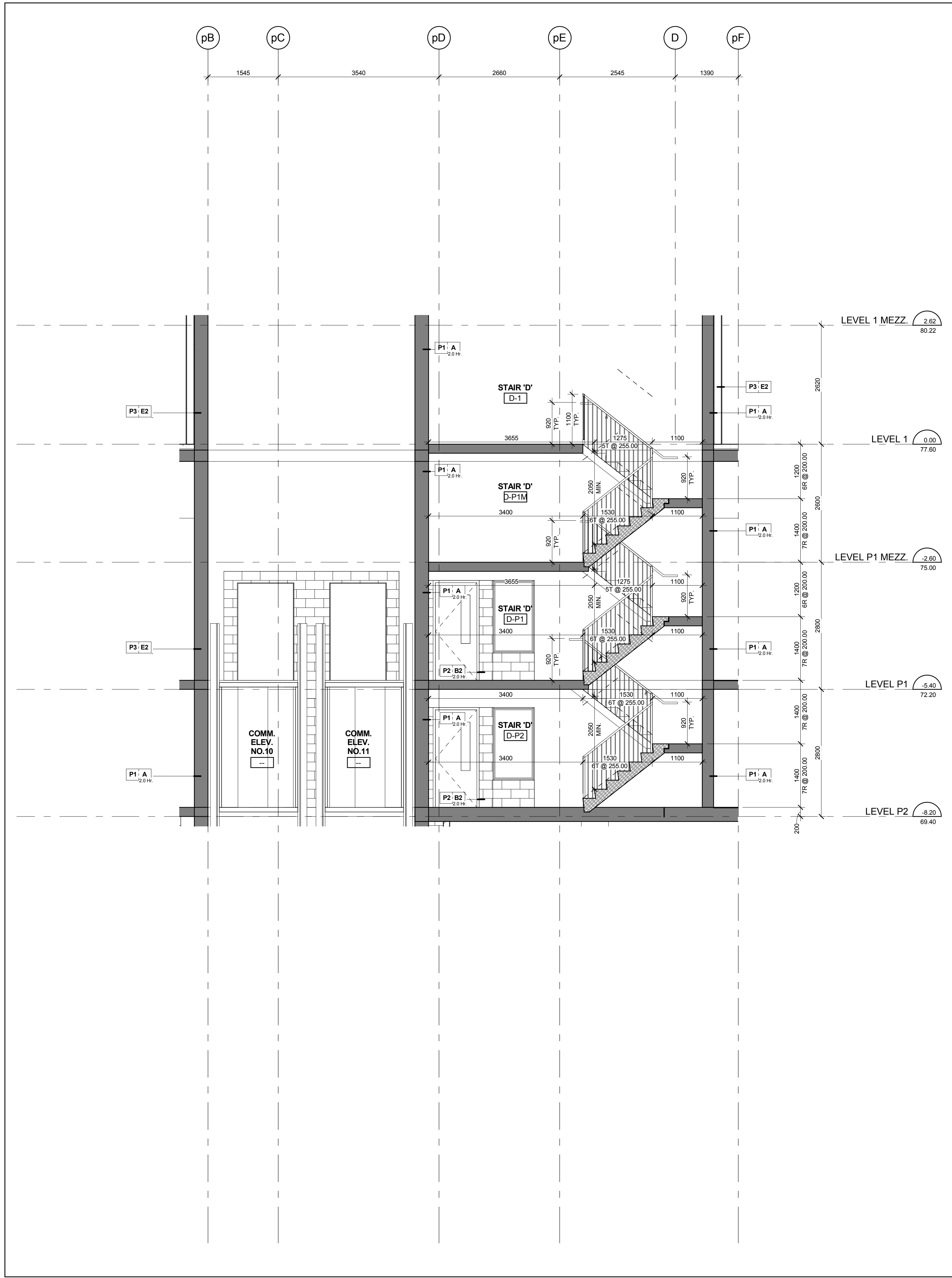
Stair 'D' - Stair Section - Levels P2 - 1 Mezzanine Scale: 1 : 50 A6-02
