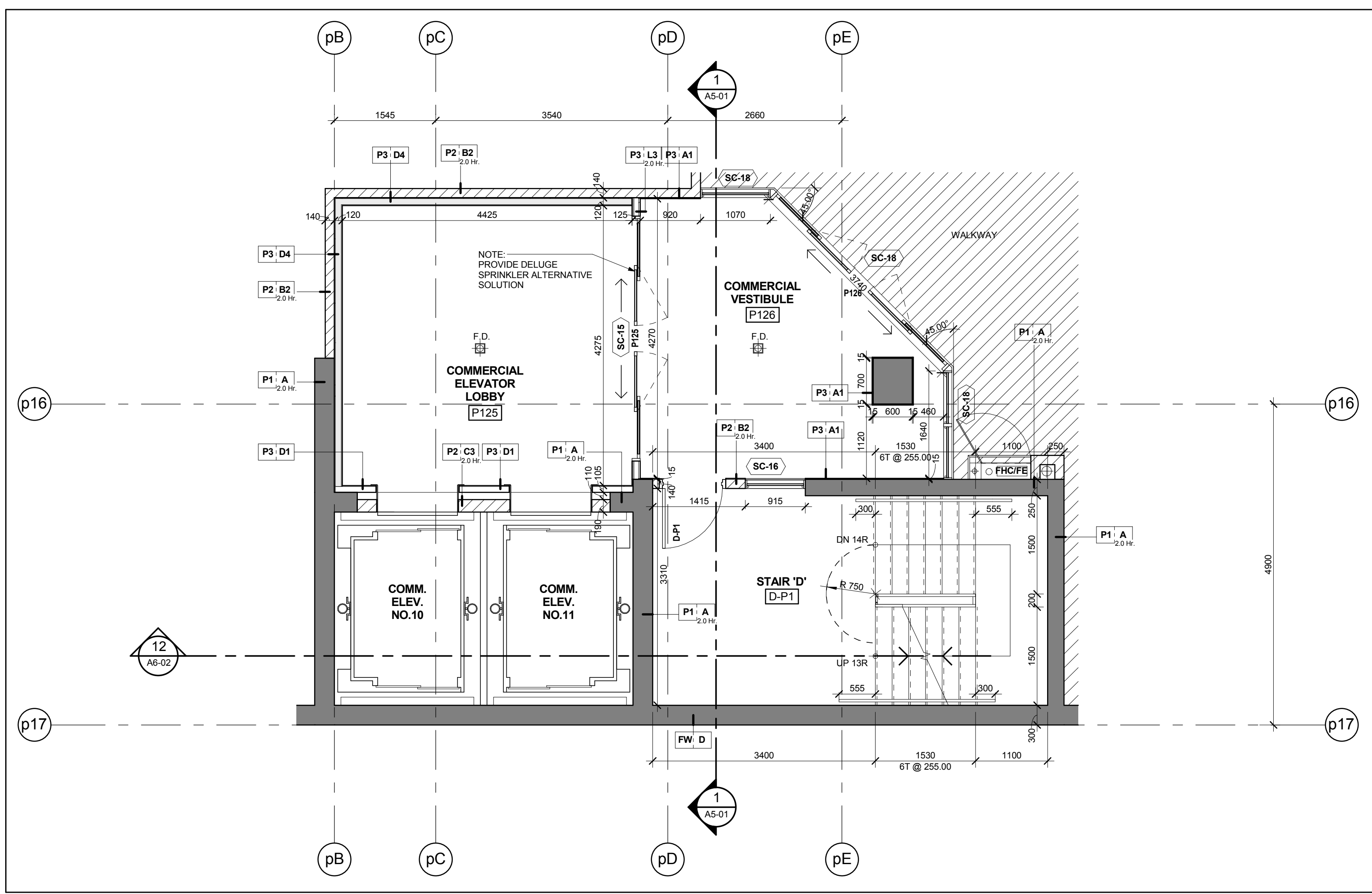
Stair 'D' - Stair Plan - Level P1 Scale: 1 : 50 A6-02
