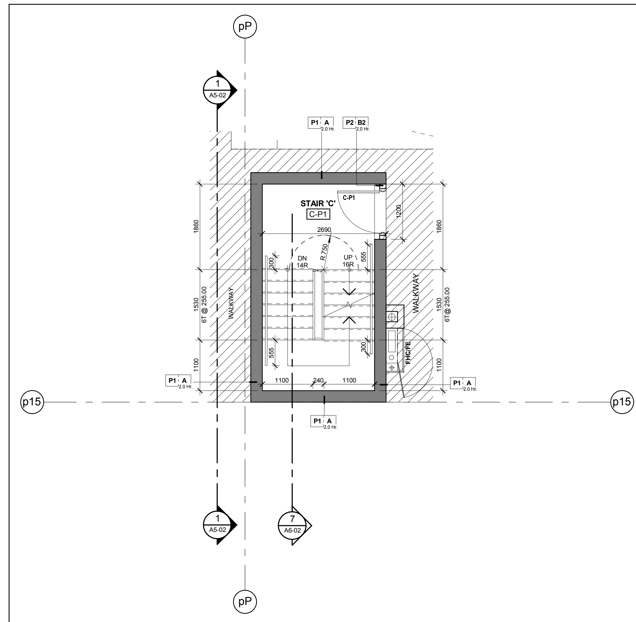
Stair 'C' - Stair Plan - Level P1 Scale: 1 : 50 A6-02
